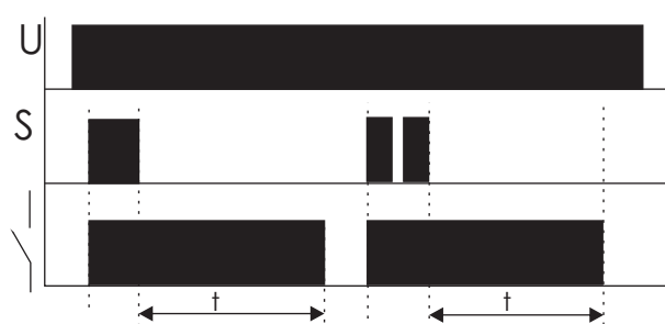
Рис.2 Диаграмма работы.
